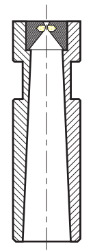
Hilera de esmaltado vertical
