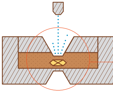
4-Pré-ouverture
