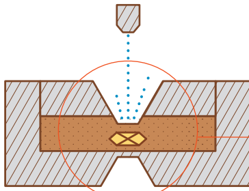
4-Preapertura
